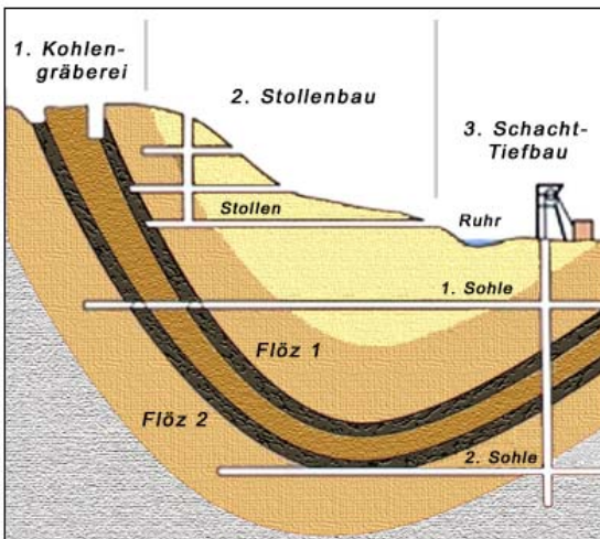
Lage der Flöz führenden Schichten im Ruhrgebiet (links Süden, rechts Norden)
